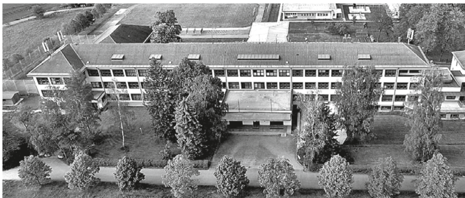
Byl zpracován projekt na výstavbu fotovoltaické elektrárny na střeše hlavní budovy ZŠ a MŠ Sedlec-Prčice
